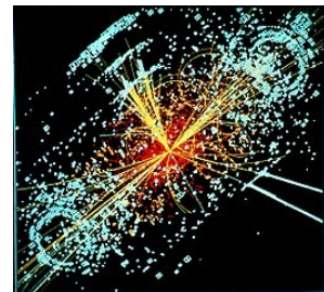
Simulation des hypothetischen Zerfalls eines Higgs-Teilchens in Teilchen-Jets am CMS/CERN; CC-BY-SA licence; Quelle , Autor: Lucas Taylor / CERN
